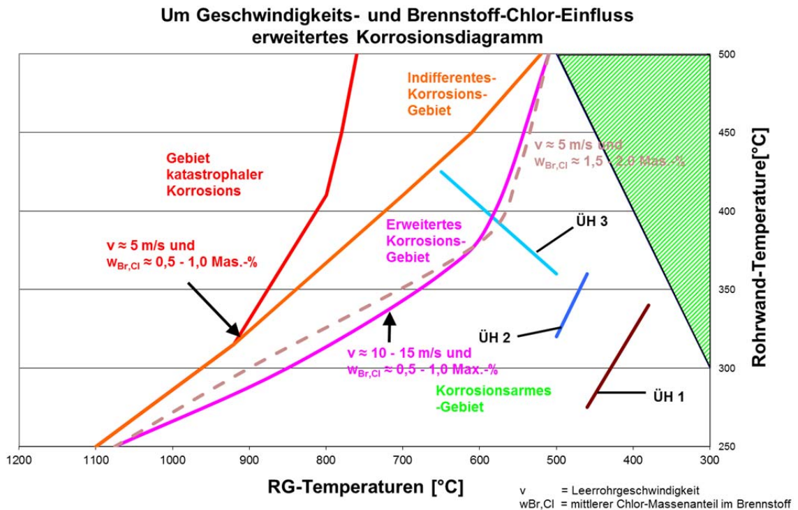
Abbildung 4.2: Um Geschwindigkeits- und Brennstoff-Chlor-Einfluss erweitertes Korrosionsdiagramm
