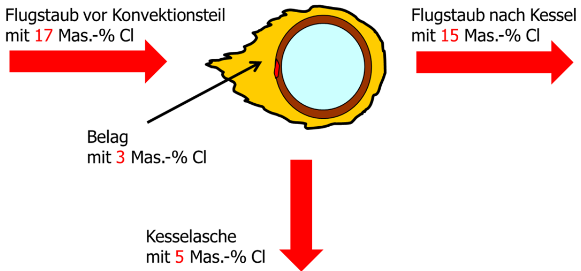
Abbildung 4.1: Chlorgehalte in der Bilanz um den Konvektionsteil eines Kessels
